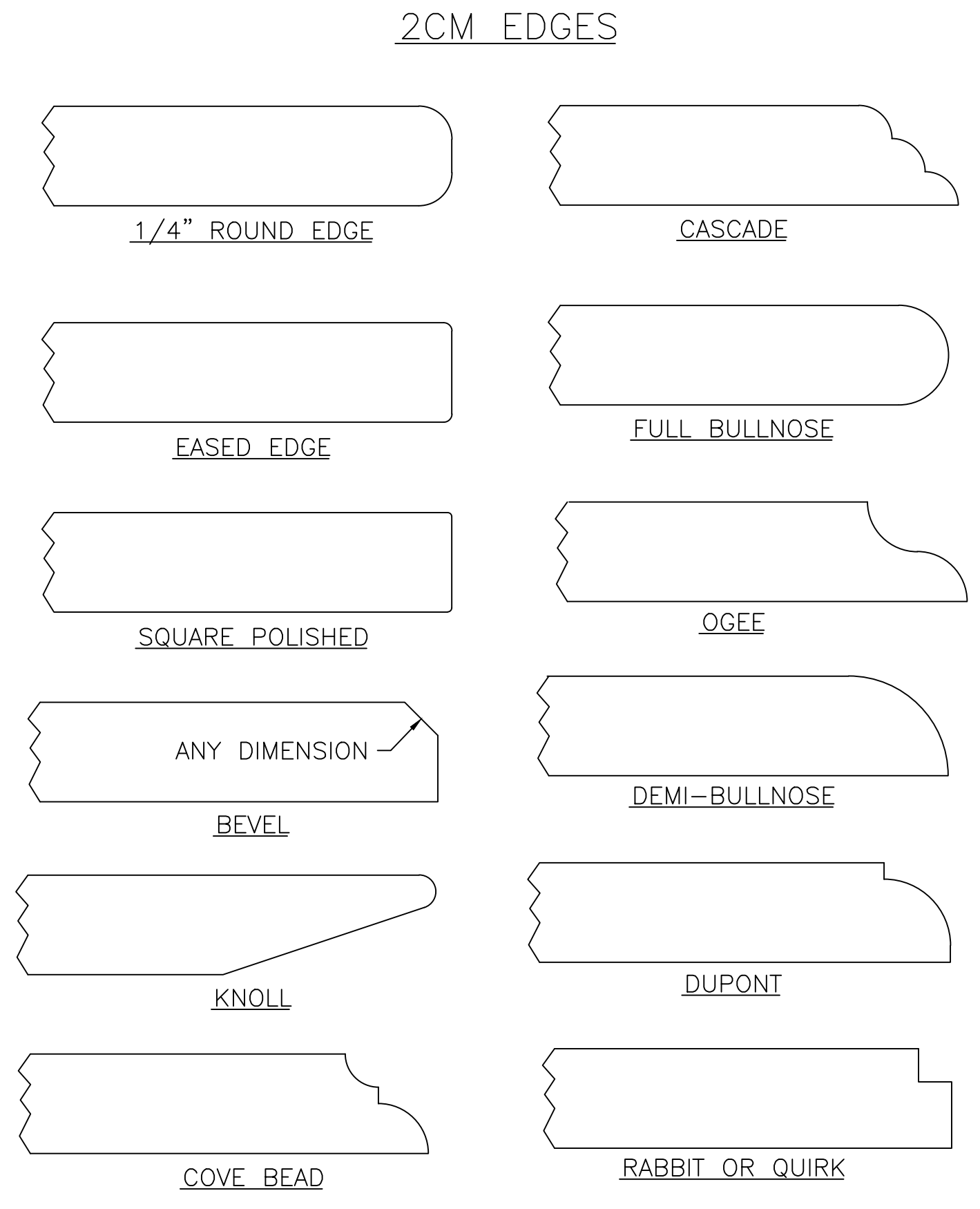
3/4" EDGE DETAILS SCALE: FULL SIZE
