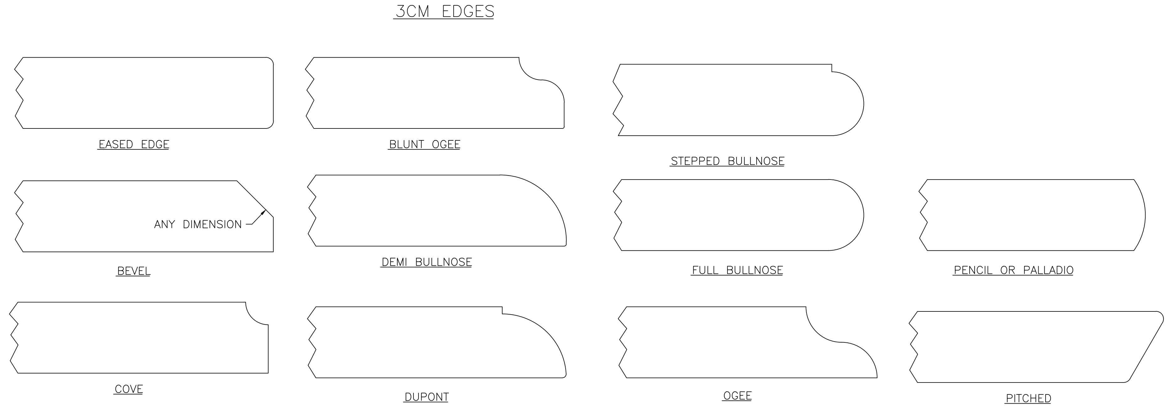
3 CM EDGE DETAILS SCALE: FULL SIZE
