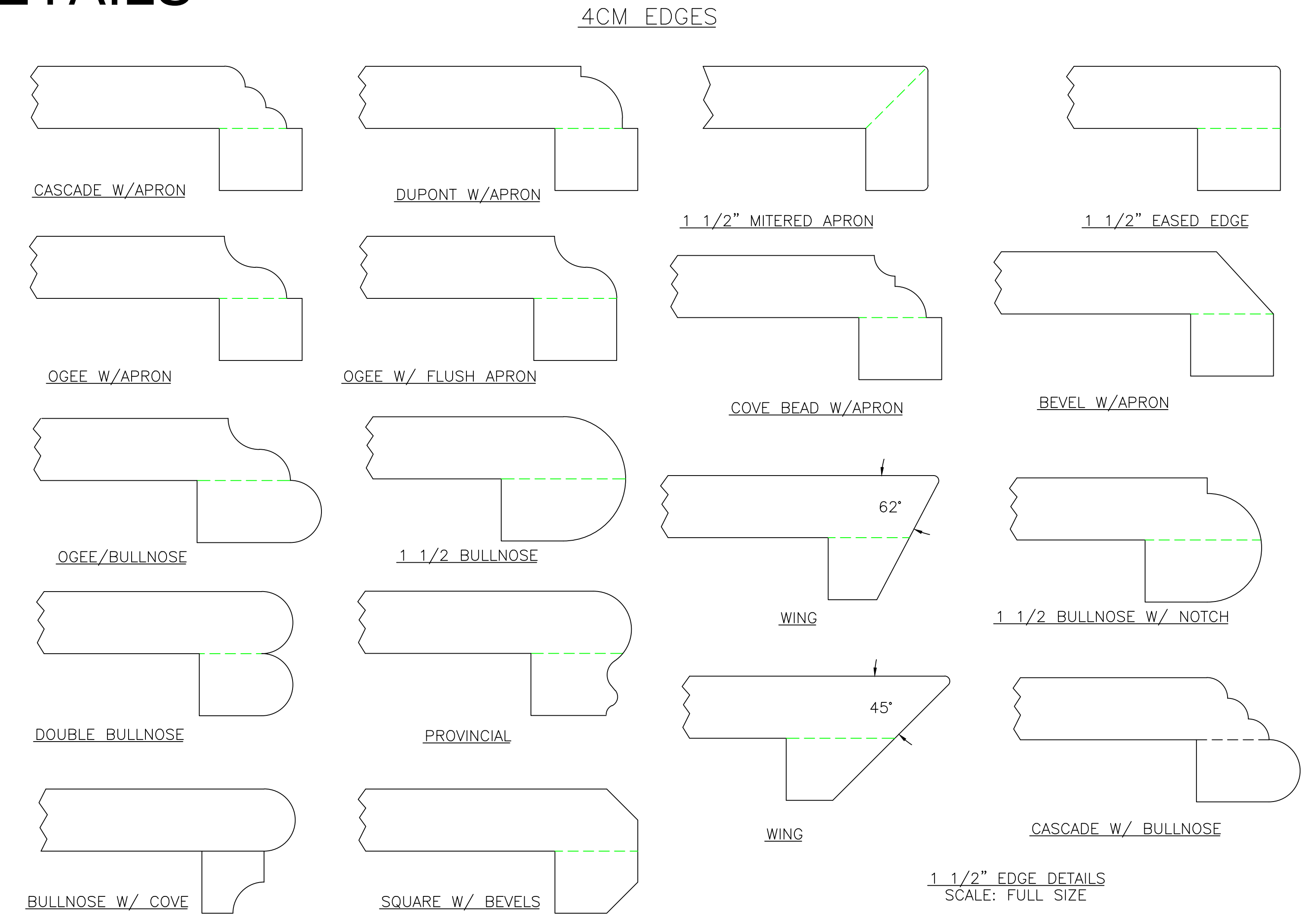
1 1/2" EDGE DETAILS SCALE: FULL SIZE
